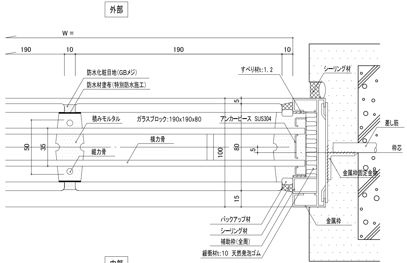
側部詳細図
