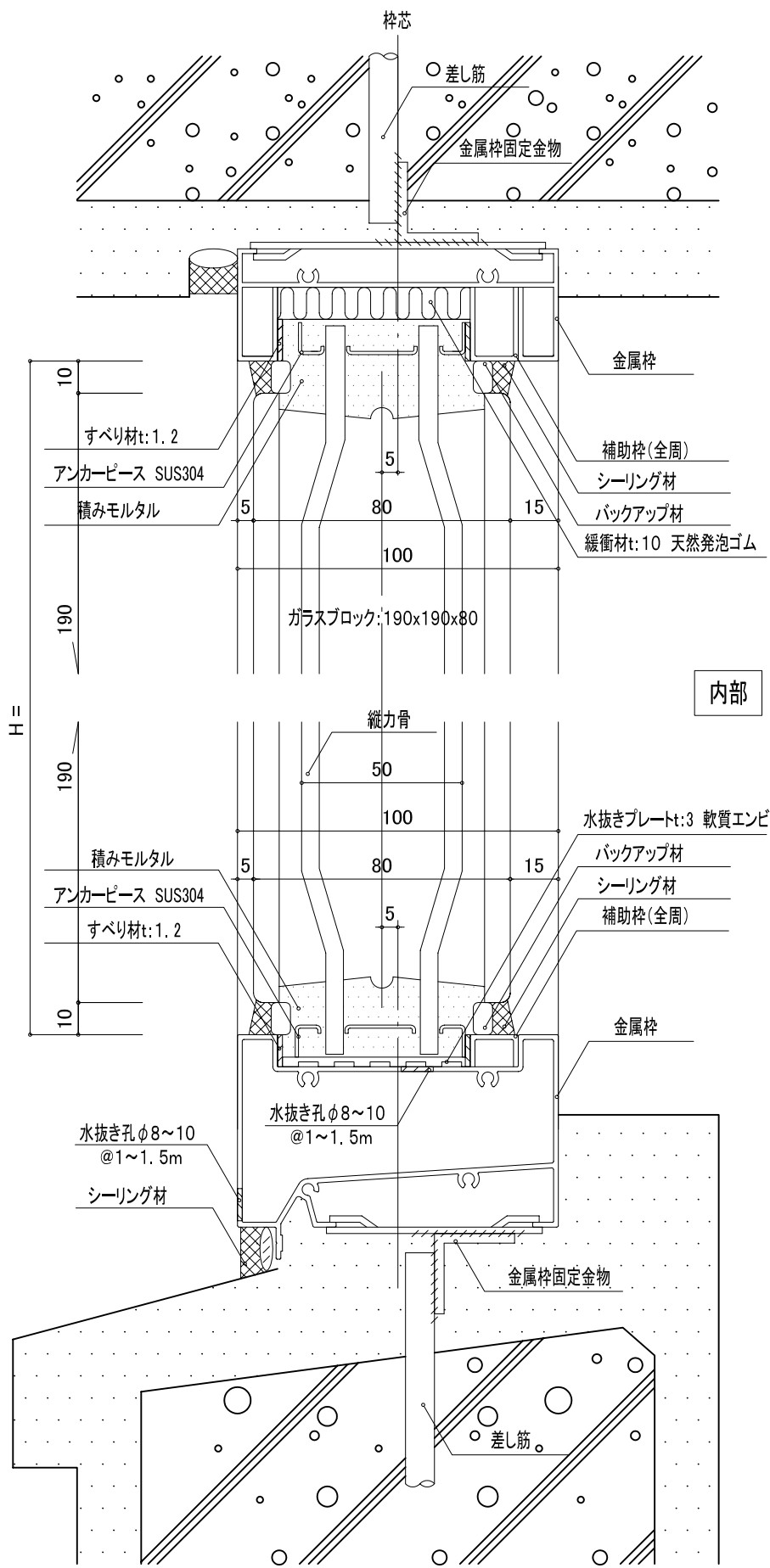
頂部詳細図
