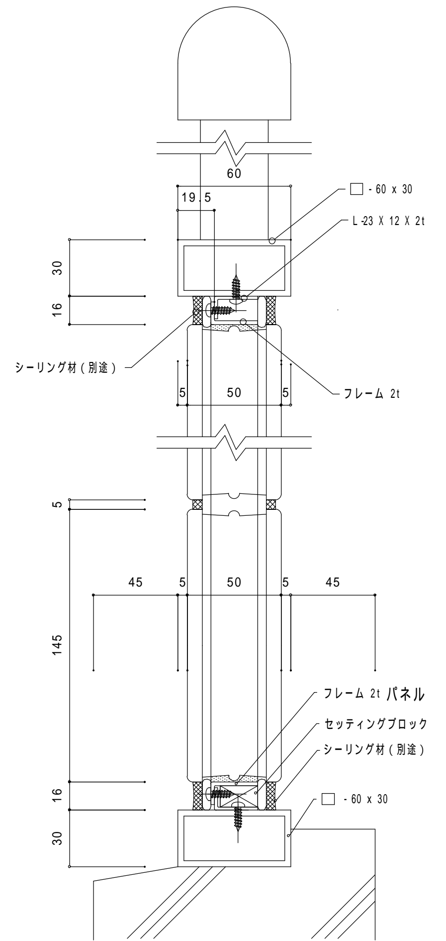
A-A断面詳細
