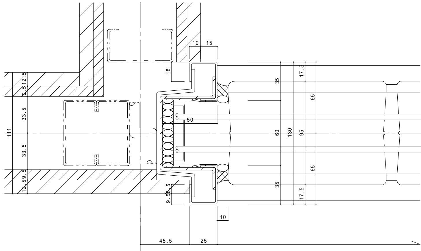
耐火間仕切壁との取り合い -1
