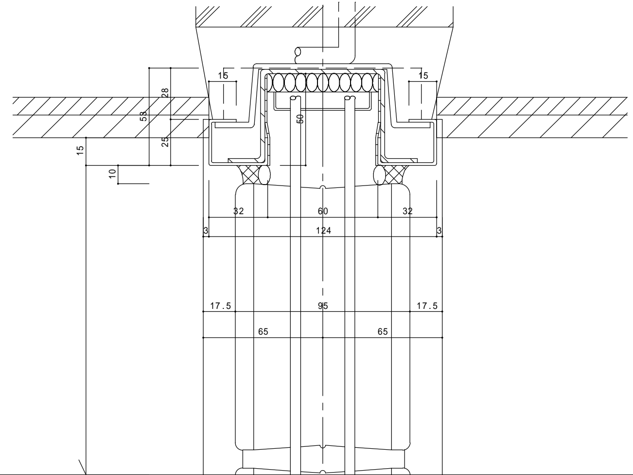
床との取り合い
