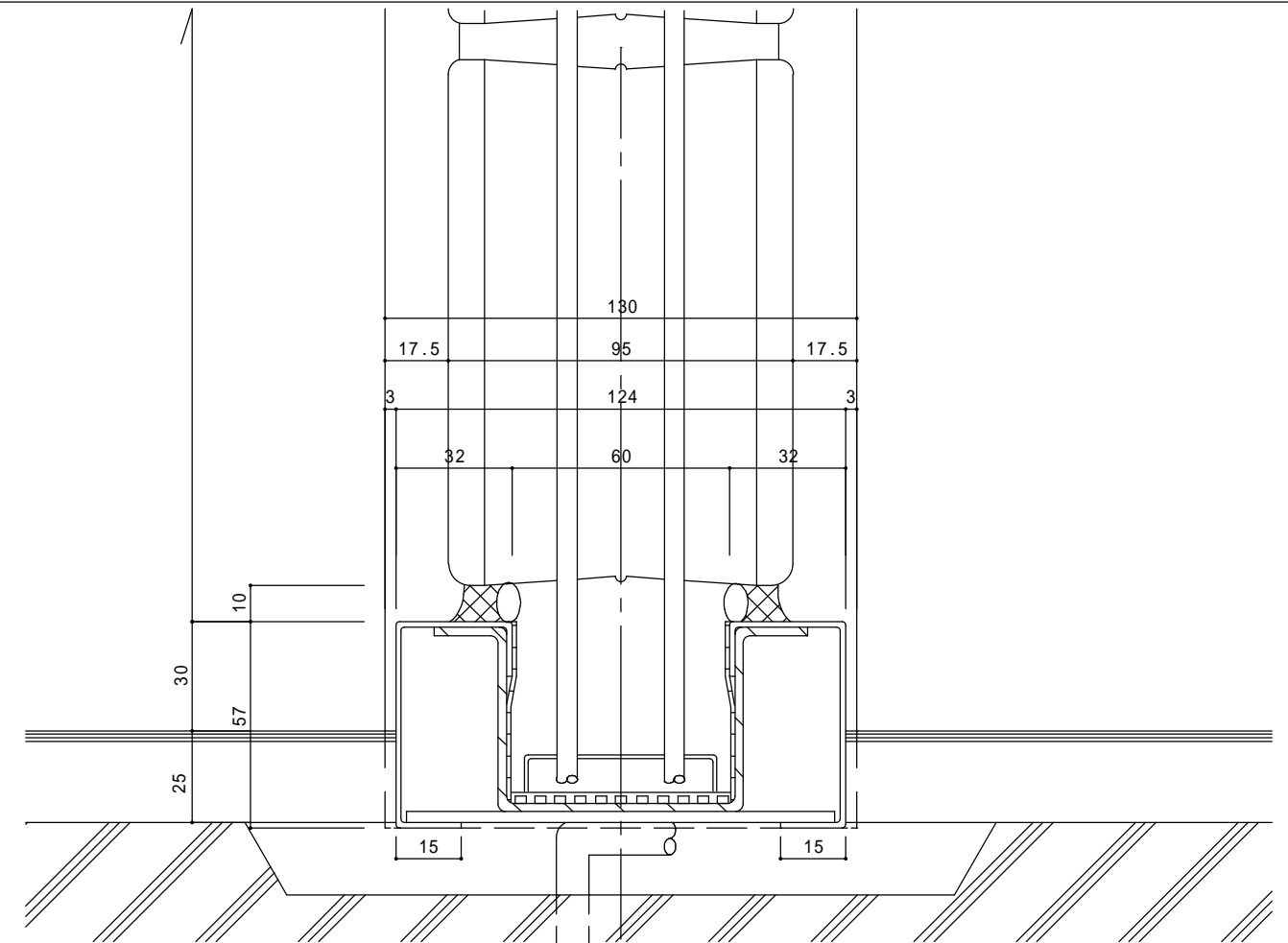
床との取り合い
