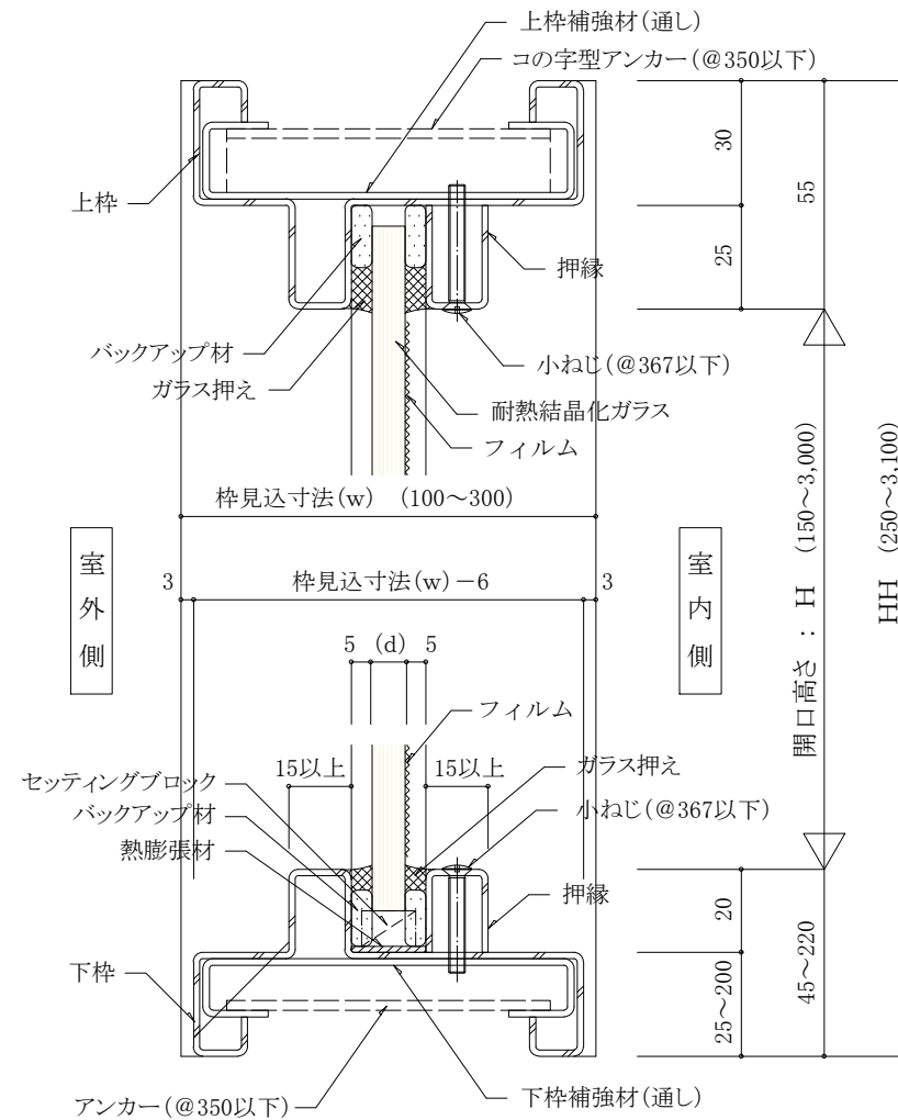
縦断面図
