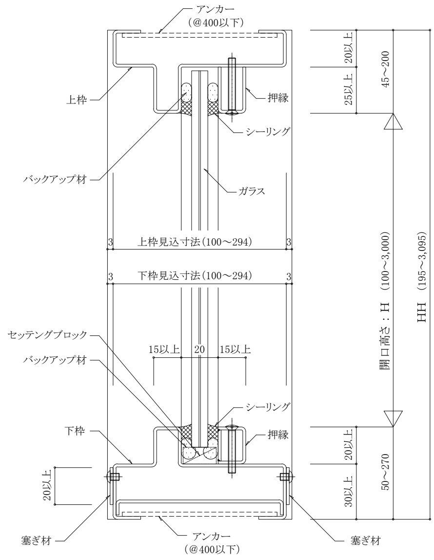
縦断面図
