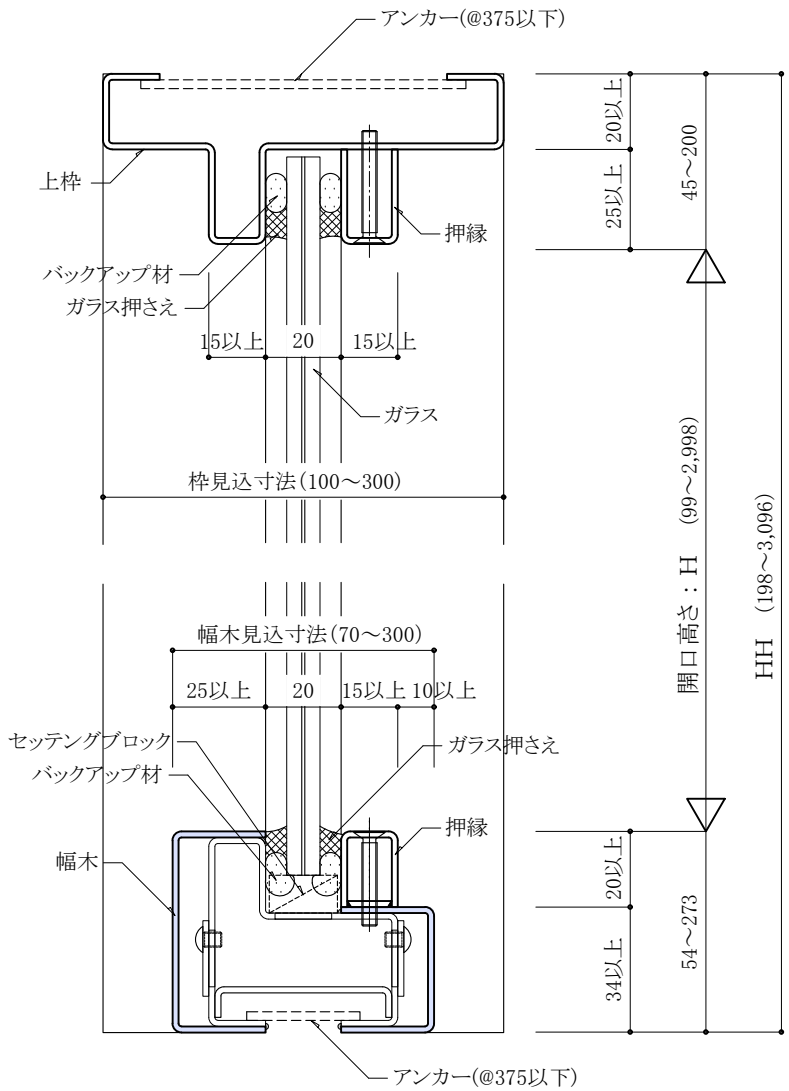
縦断面図
