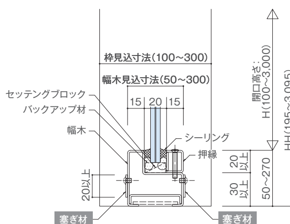
縦断面図（幅木タイプ）
