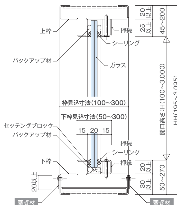
縦断面図
