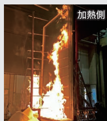
加熱側 火源上部の最高温度は約800℃
