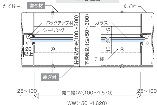
水平断面図
