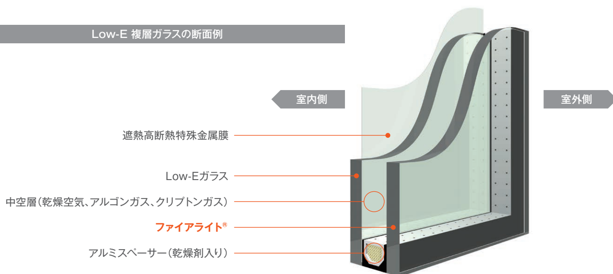
Low-E トリプルガラスの断面例
